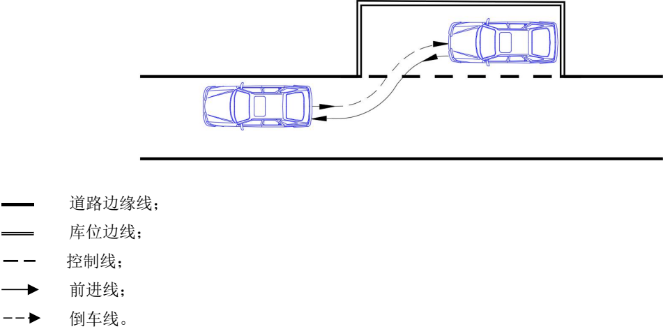
图7 侧方停车考试车辆运行路线图
