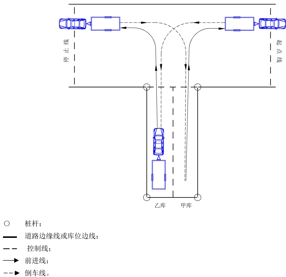
图4 轻型牵引挂车准驾车型桩考车辆运行路线图
