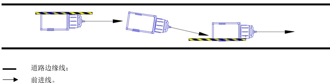
图 9 三轮汽车、普通三轮摩托车通过单边桥考试车辆运行路线图
